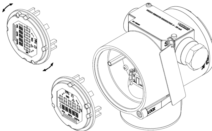
Figura 2.4 – Rotação do Display Digital LCD 4 x 90°.
