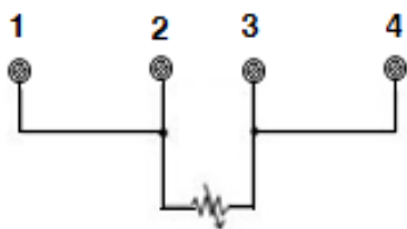
Figura 2.8 - Conexão RTD ou resistivos a 2 fios.
