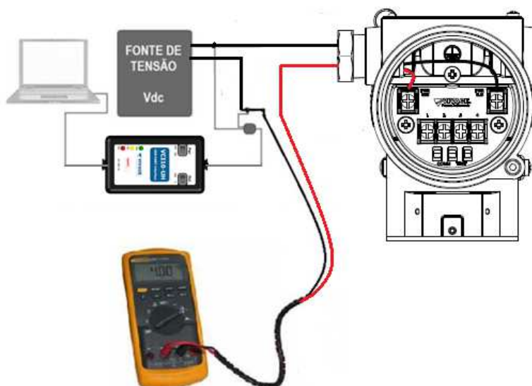
Figura 3.10 – Esquema de montagem para o Trim de corrente do VTT10-FH.
