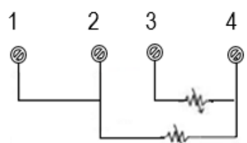
Figura 2.11 - Conexão RTD ou resistivo diferencial, máximo, mínimo e backup.
