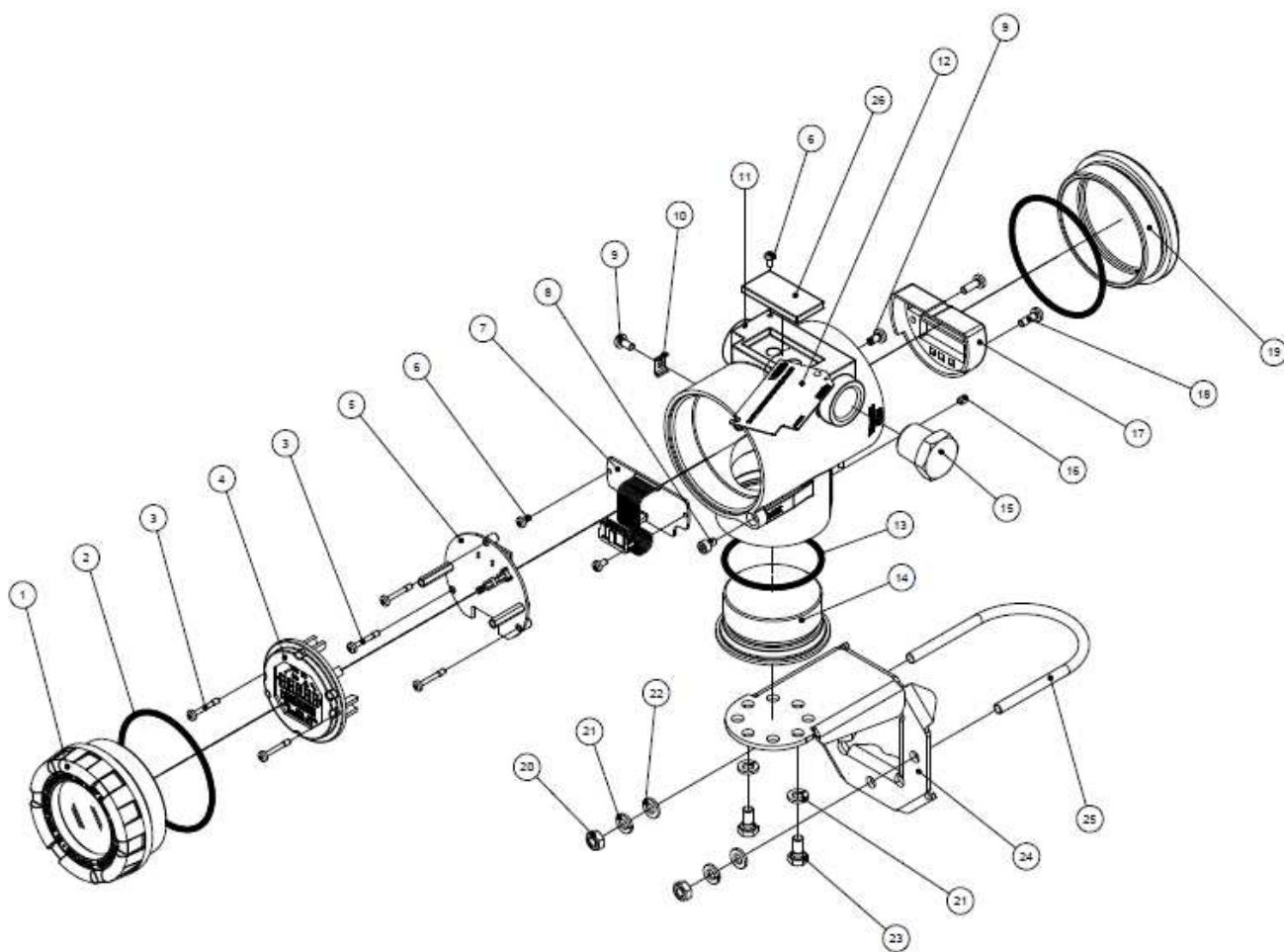
Figura 4.1 – Desenho explodido do VTT10-FH.
