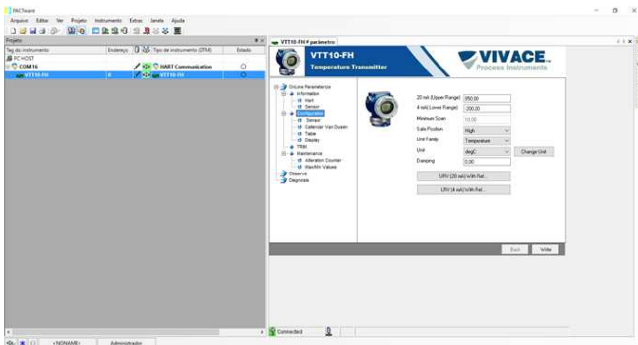
Figura 3.11 – Tela de configuração da faixa de trabalho do VTT10-FH no PACTware.
