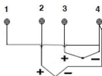
Figura 2.13 - Conexão termopar ou mV diferencial, máximo, mínimo e backup.
