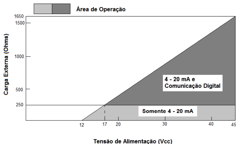
Figura 3.8 – Curva de carga do VTT10-FH.
