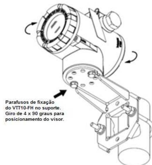
Figura 2.3 – Ajuste da posição da carcaça.
