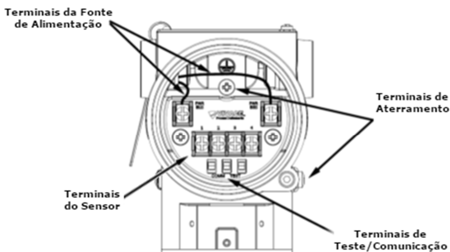
Figura 2.6 – Conexões e descrição dos terminais do VTT10-FH.
