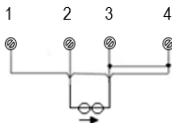
Figura 2.14 - Conexão entrada 4 - 20 mA.
