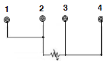
Figura 2.9 - Conexão RTD ou resistivos a 3 fios.
