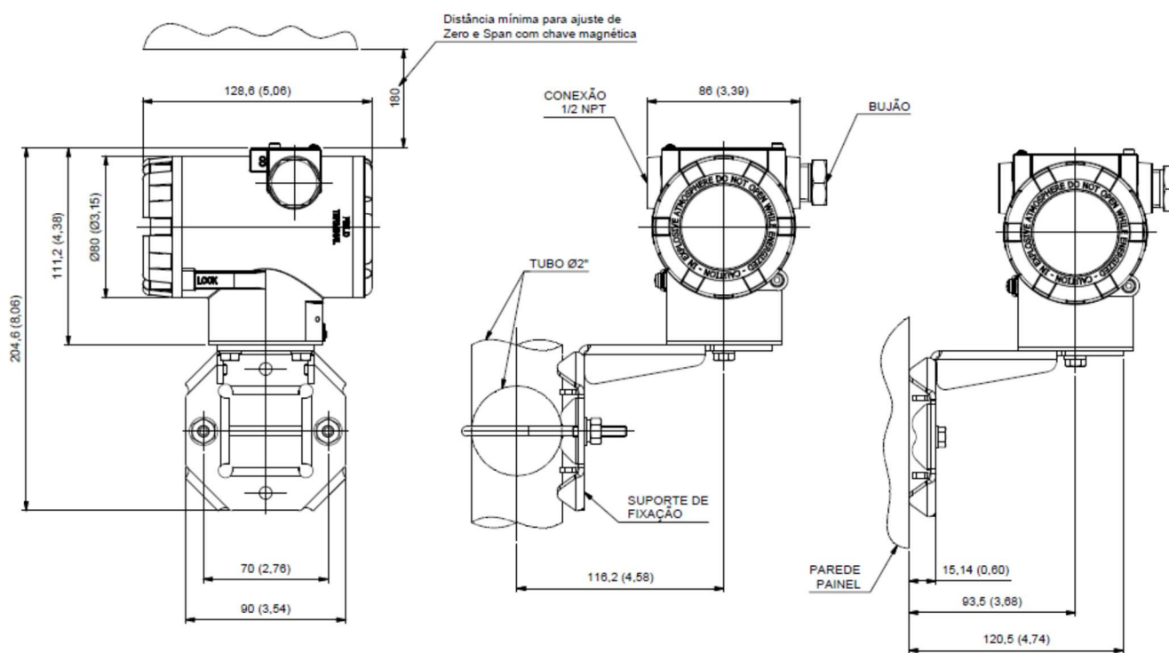
Figura 2.1 – Desenho dimensional e esquema de montagem do VTT10-FH.
