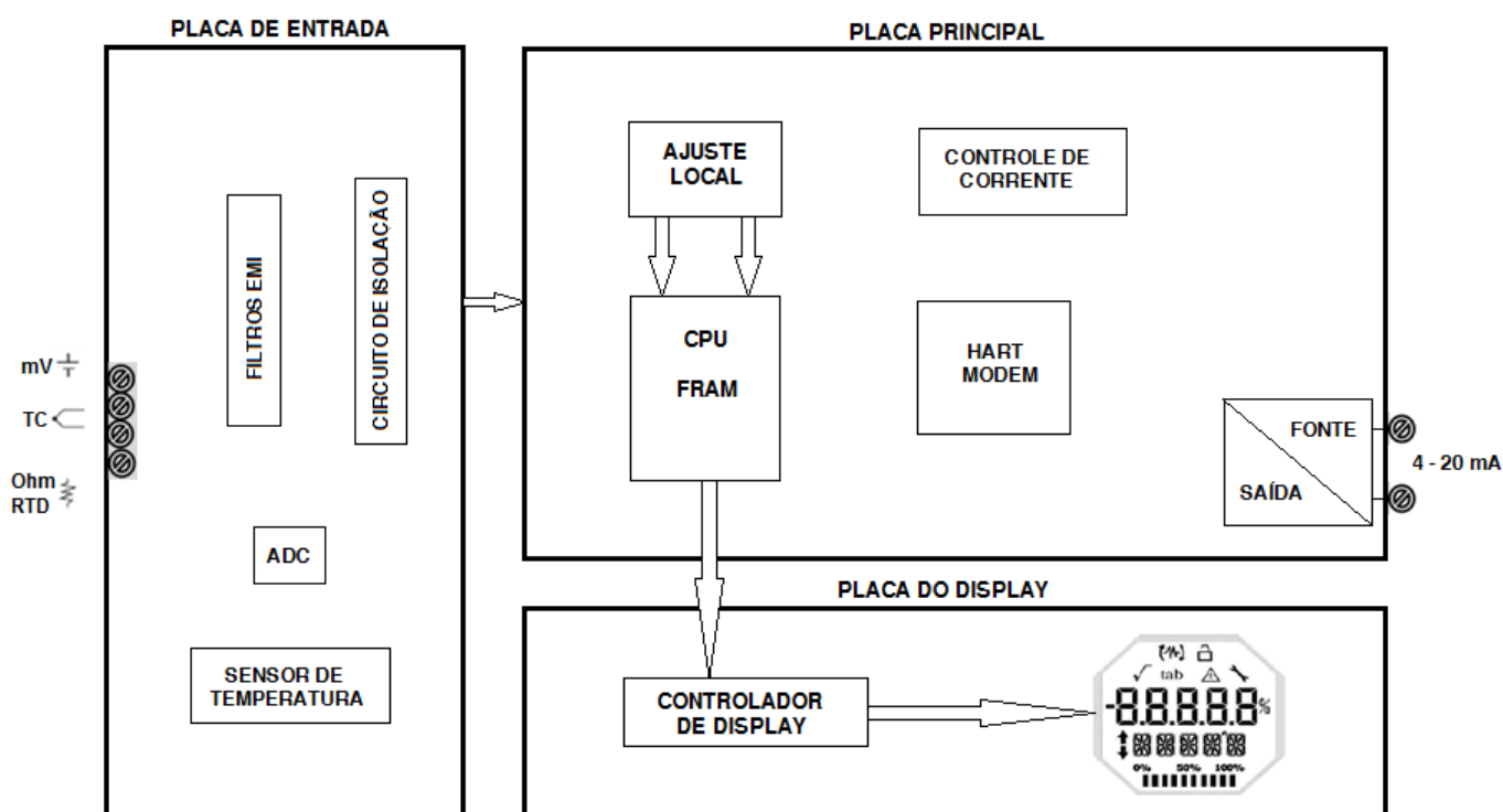
Figura 1.1 - Diagrama de blocos do VTT10-FH.
