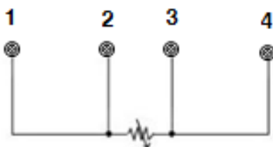
Figura 2.10 - Conexão RTD ou resistivos a 4 fios.
