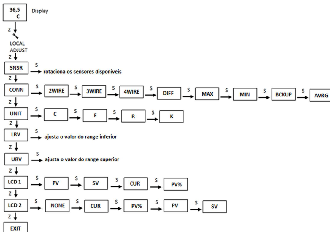
Figura 3.4 – Árvore de programação do ajuste local.
