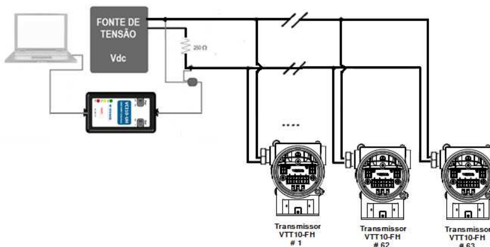
Figura 3.7 – Esquema de ligação da interface ao VTT10-FH em configuração multidrop.
