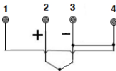
Figura 2.12 - Conexão termopar ou mV.
